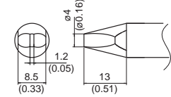
TX2-XBCR6 Shape-6XBCR
