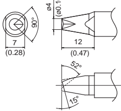
TX1-XDR3 Shape-3XDR
