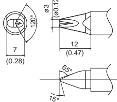
TX1-XDR3 Shape-3XDR
