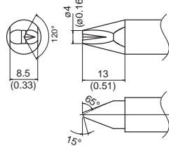
TX2-XDR4 Shape-4XDR
