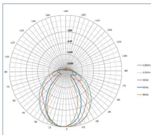
Vertical Pattern HyperLOG 30xx Serie
