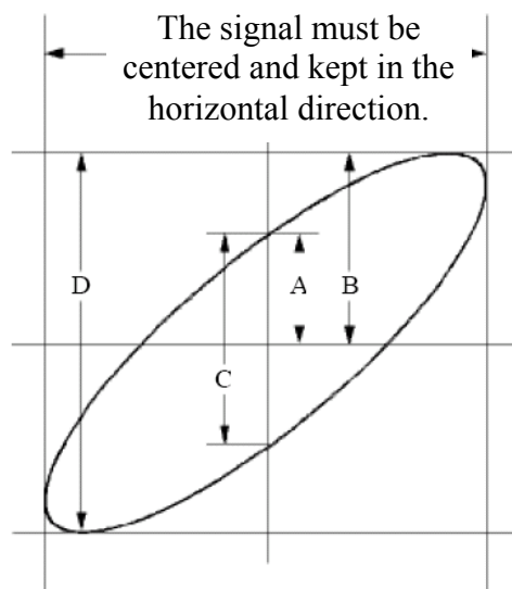
Fig.6-6 Lissajous Graph
