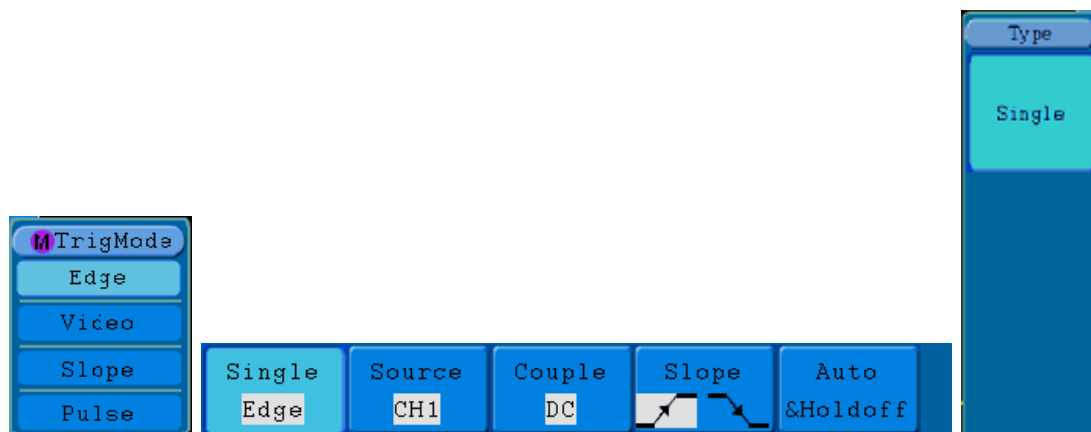
Figure 30. Edge trigger menu.
