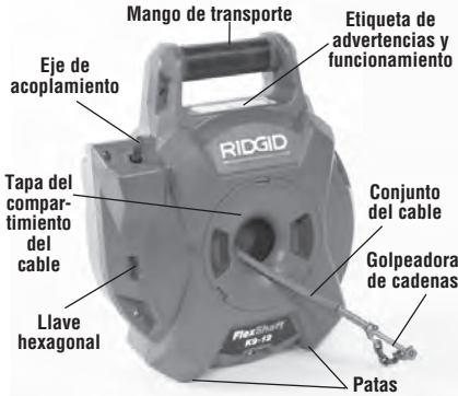
Figura 1 A – Limpiadora de desagües FlexShaft K9-12 de RIDGID®
