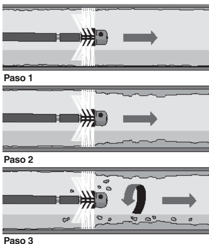
Figura 17 – Limpieza de las paredes del desagüe con una escobilla
