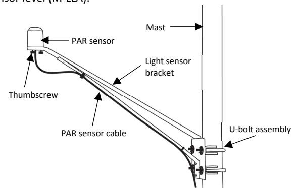
PAR Sensor Bracket Mounting
